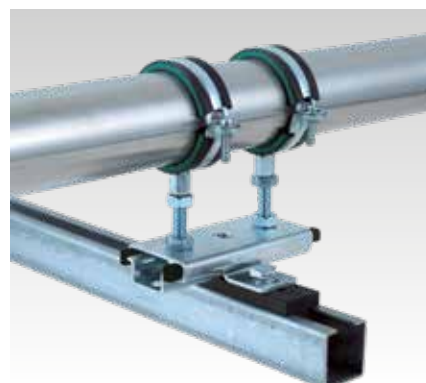
Montage von einem Gleitkörper und Schiebeschlitten, stehend auf einer MPC-Systemschiene
