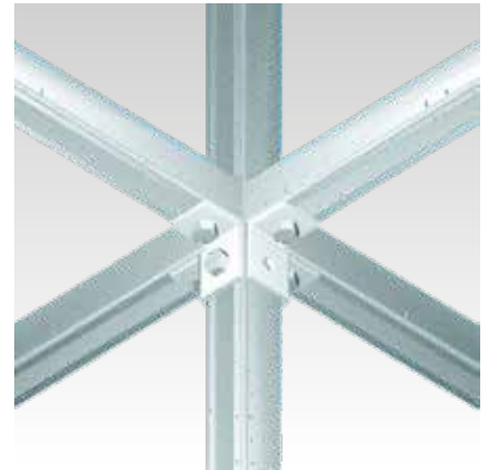
Regalbau aus MPC-Systemschienen- Knotenpunkt mit Abgang in 4 Richtungen
