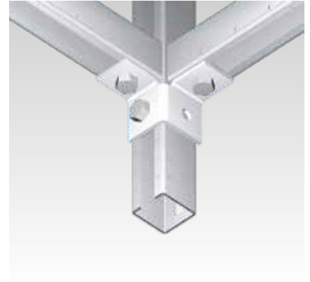
MPC-Seitenwinkel beidseitig
