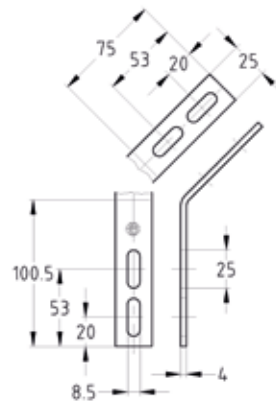
Montagewinkel 45°
